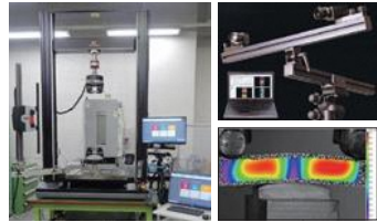
万能材料試験機<30kN>
