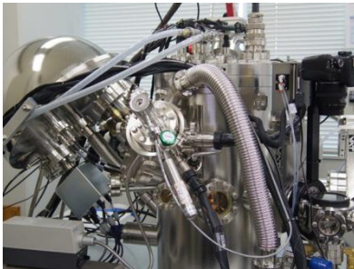
X線光電子分光分析装置
