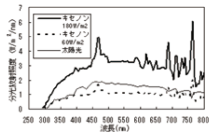
図 キセノンランプの分光分布 (岩崎電気株式会社テクニカルレポートより)
