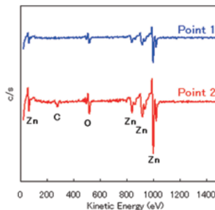
オージェ電子分光分析結果
